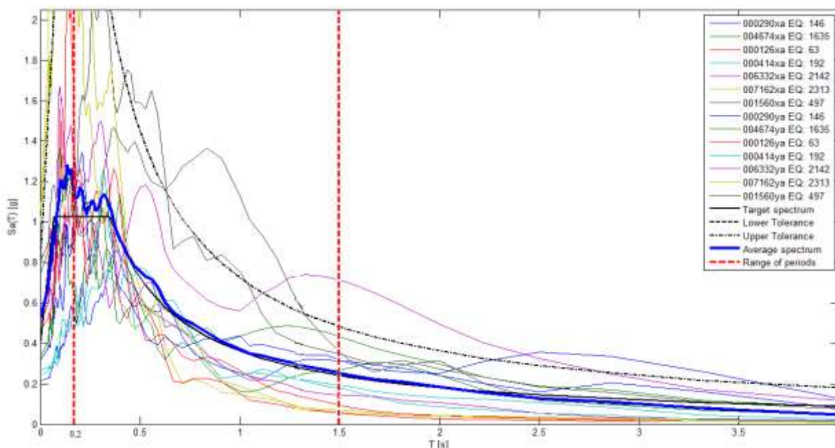
الشكل (11): متوسط أطياف المجموعة الأولى (14 مركبة لسبعة زلازل) في مجال الدور قيد الاهتمام للدور T = 1 \text{ sec} .
