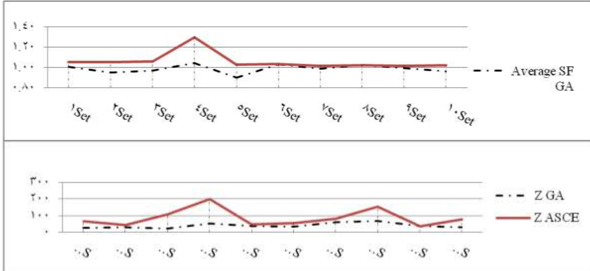
الشكل (13): تغير المتوسط الحسابي لمعاملات التقييم لكل مجموعة والنتيجة عن التقييم باستخدام الطريقتين GA ، ASCE، وتغير مربع المساحة المحصورة بين الطيف المتوسط والطيف الهدف لكل مجموعة والنتائج عن التقييم باستخدام الطريقتين.
