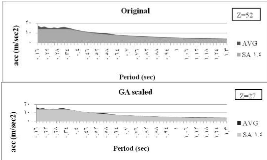
الشكل (12): متوسط أطياف الاستجابة AVG والطيف الهدف 1.4 SA في مجال الدور قيد الاهتمام لكل من السجلات الأصلية والمقيسة بطريقة الخوارزمية الجينية للمجموعة الأولى فقط على مجال الدور (0.2-1.5).
